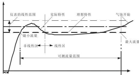
图1.1 涡轮流量计特性曲线
