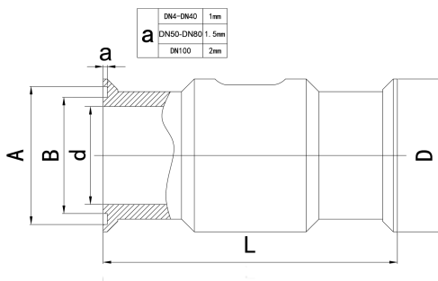
卫生型涡轮传感器外形尺寸图
