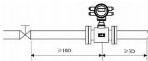
图 10 阀门位于传感器上游的安装
